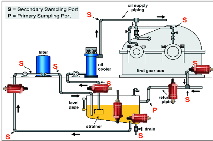
[기어박스(강제 순환식)]
